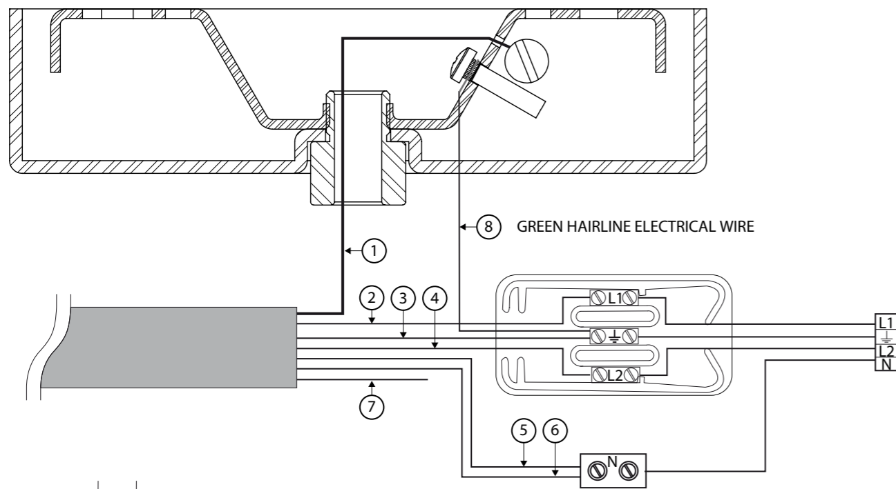
schema elettrico - wiring diagram - schaltplan - schéma de câblage - diagrama de cableado
